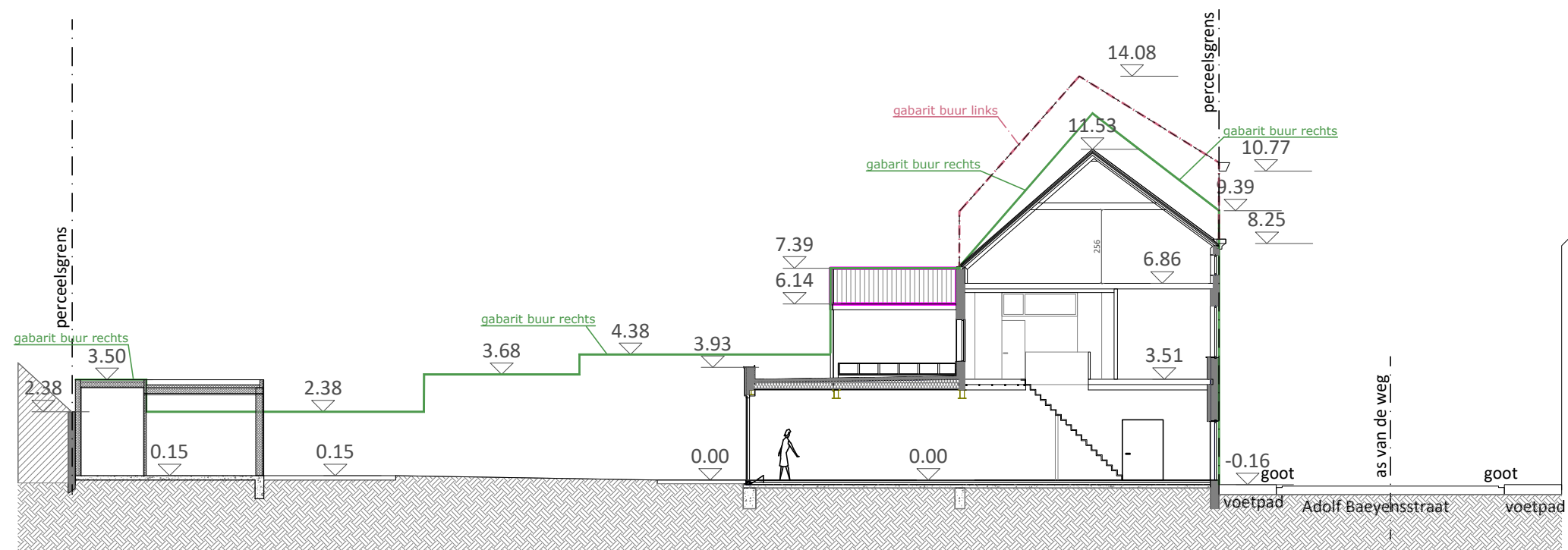
BESTAANDE TOESTAND TERREINPROFIEL B-B schaal 1-200
