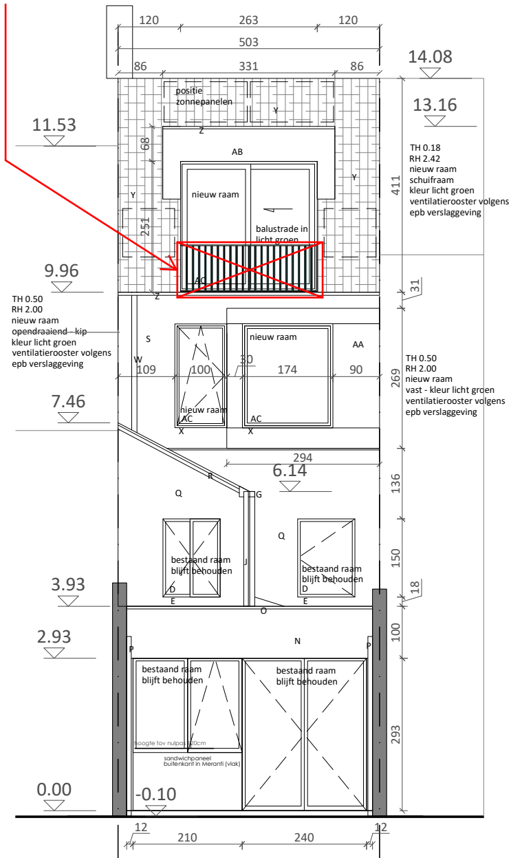
NIEUWE TOESTAND ACHTERGEVEL schaal 1-100
