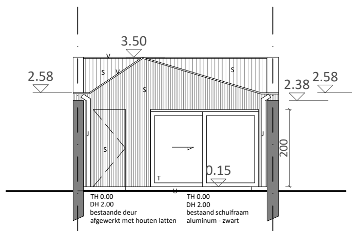
BESTAANDE TOESTAND GEVEL tuin atelier schaal 1-100
