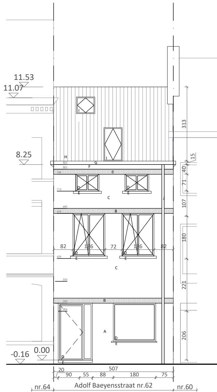
BESTAANDE TOESTAND VOORGEVEL schaal 1-100
