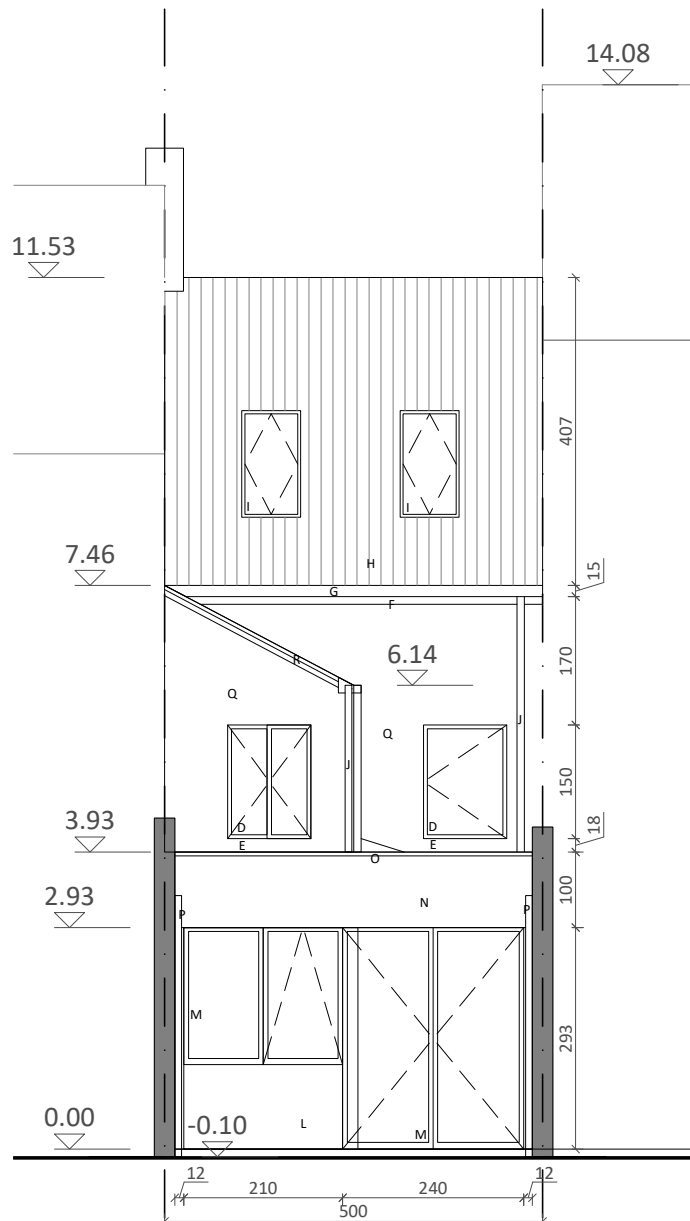
BESTAANDE TOESTAND ACHTERGEVEL schaal 1-100
