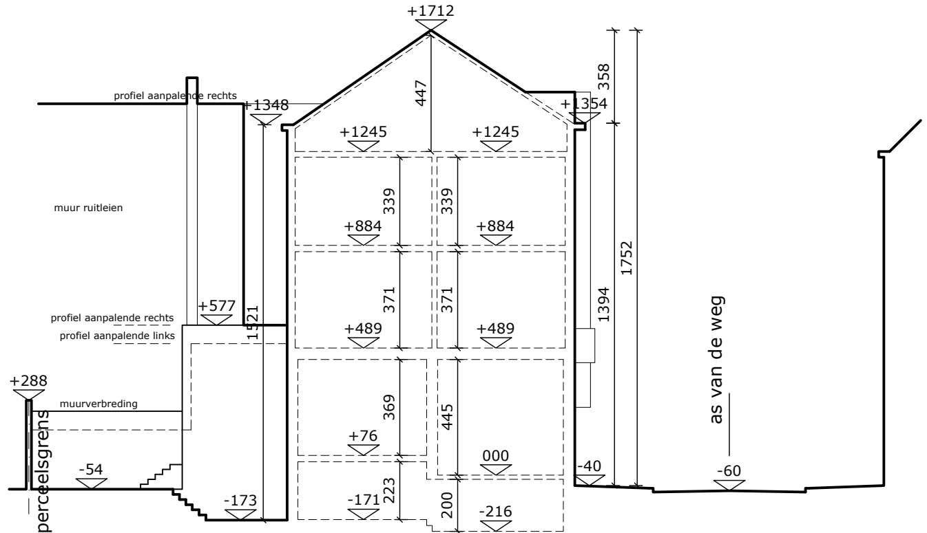
TERREINPROFIEL T2 (rechts) - schaal 1/200
