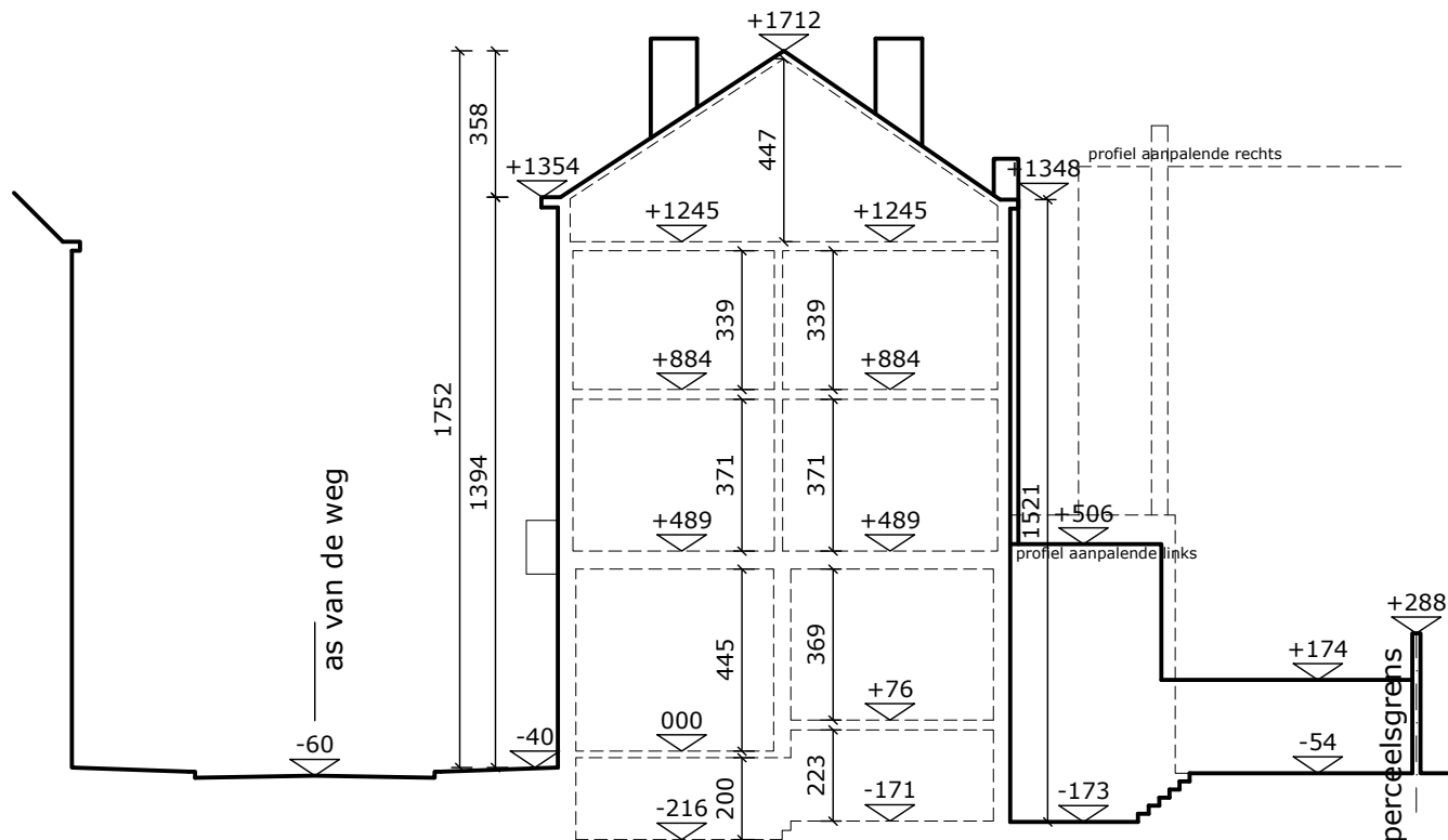
TERREINPROFIEL T1 (links) - schaal 1/200
