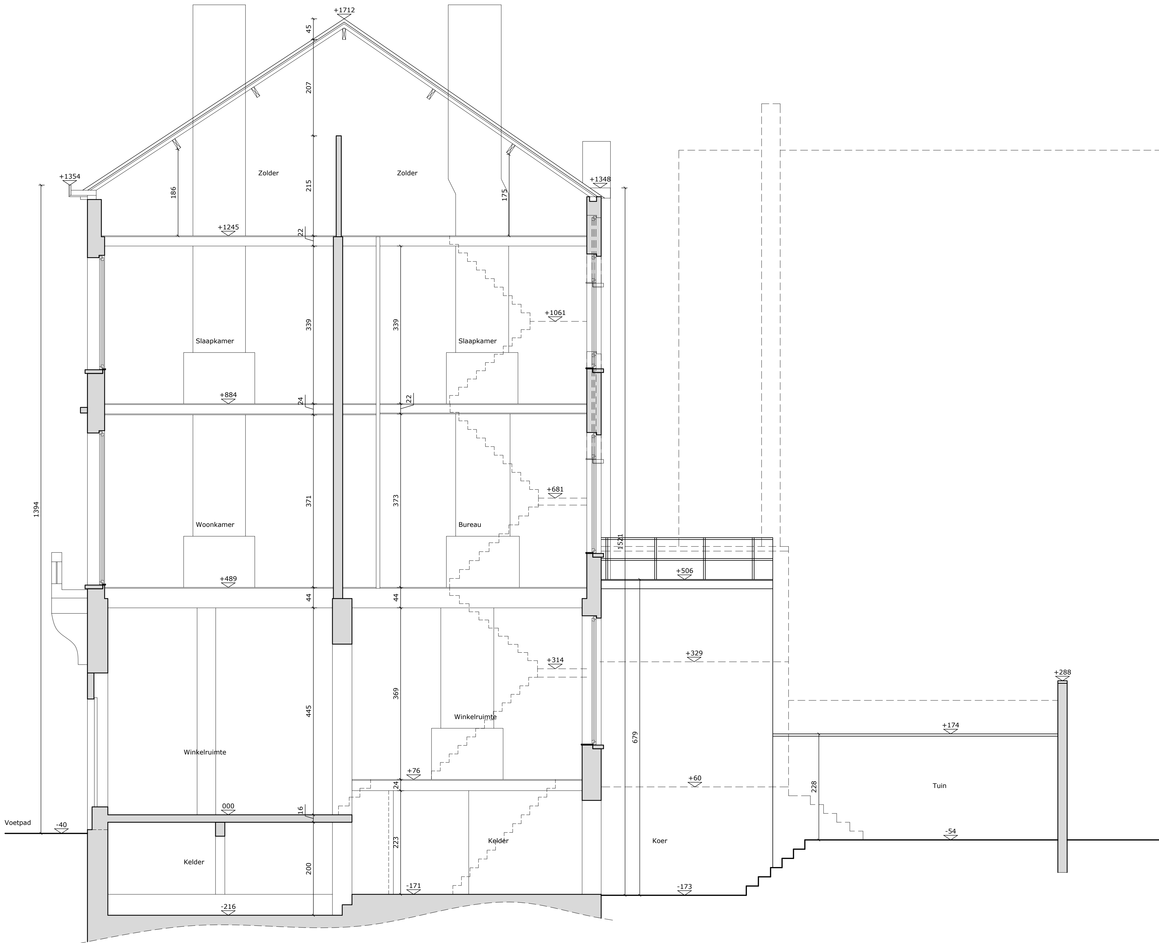
SNEDE A AFMETINGEN OP PLAN IN CENTIMETER bestaande toestand - 1/50
