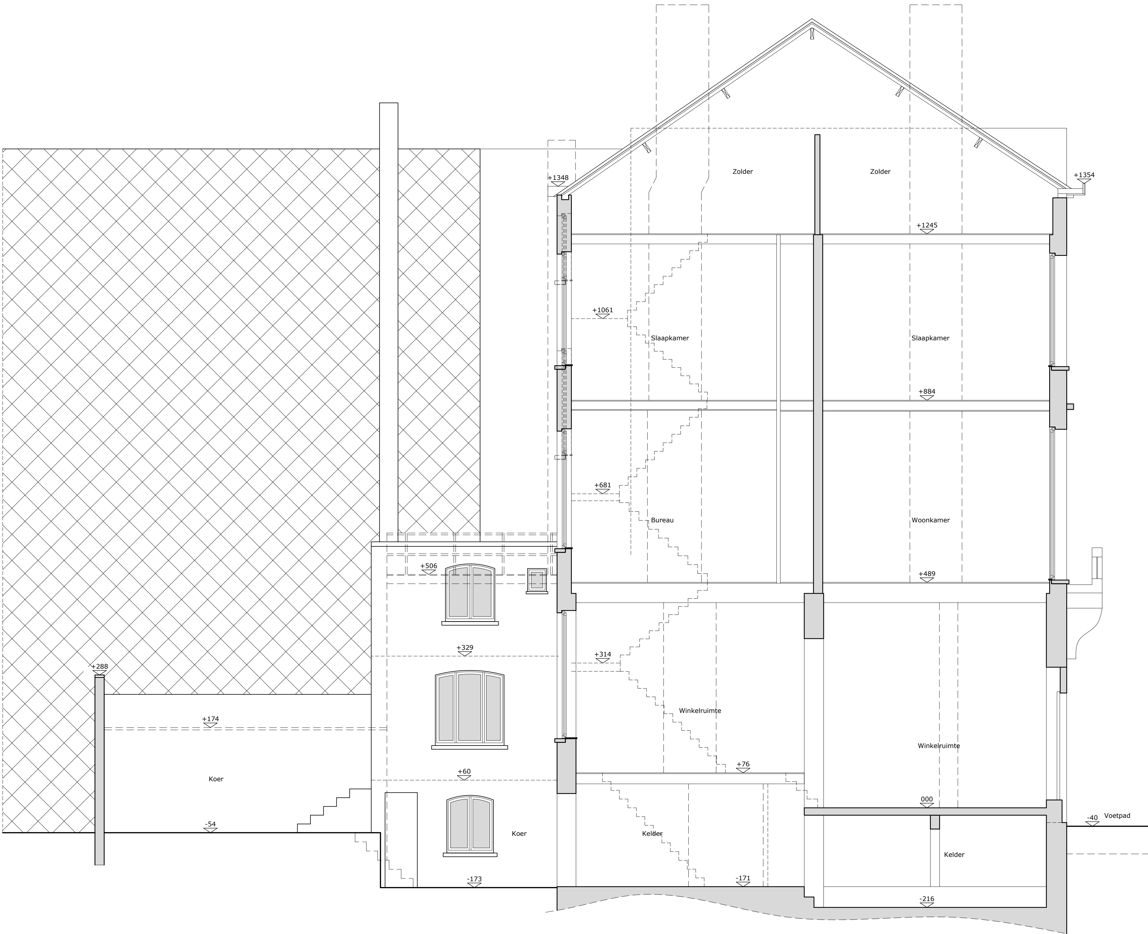
SNEDE B AFMETINGEN OP PLAN IN CENTIMETER bestaande toestand - 1/50
