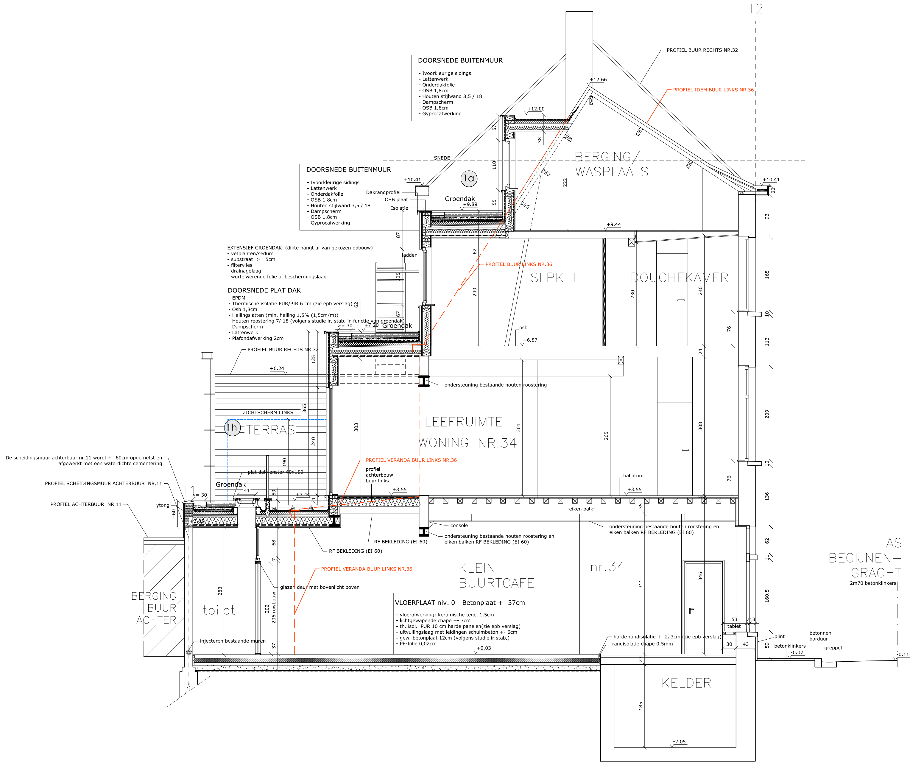
DOORSNEDE AA' / TERREINPROFIEL T1 - T2
