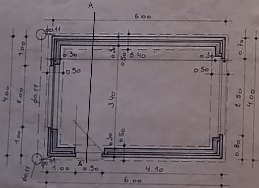
grondplan. fundering
