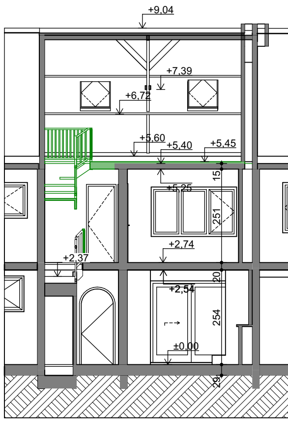
N S Doorsnede A-A 1:100
