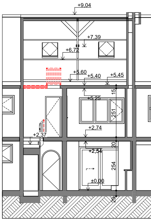
S. B Doorsnede A-A 1:100
