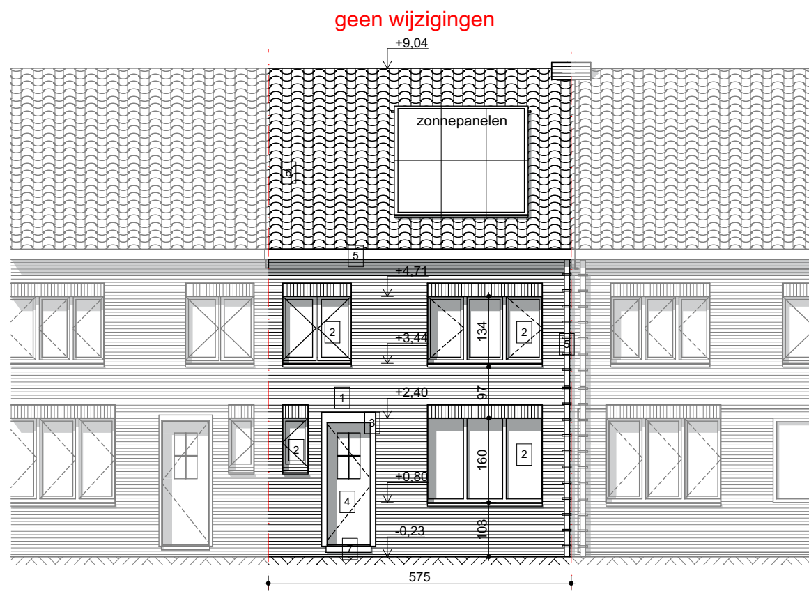
G_N Voorgevel 1:100
