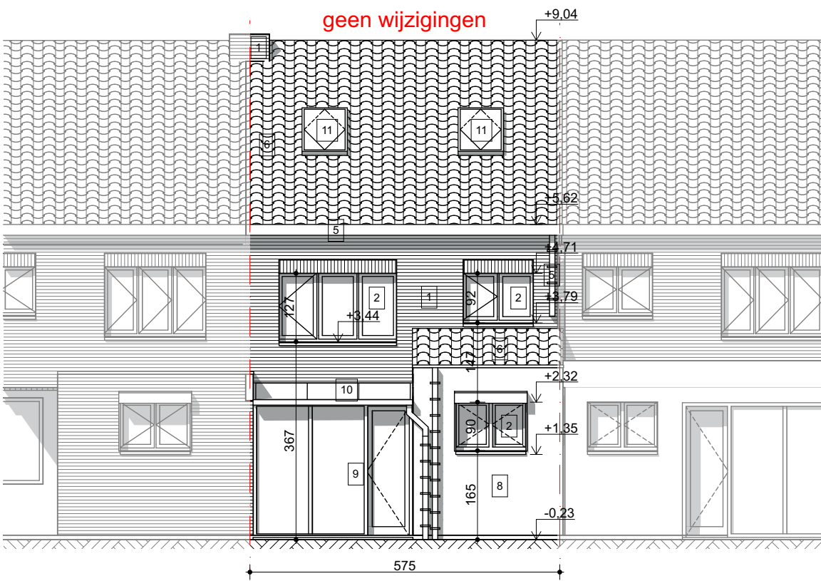
G_B Achtergevel 1:100
