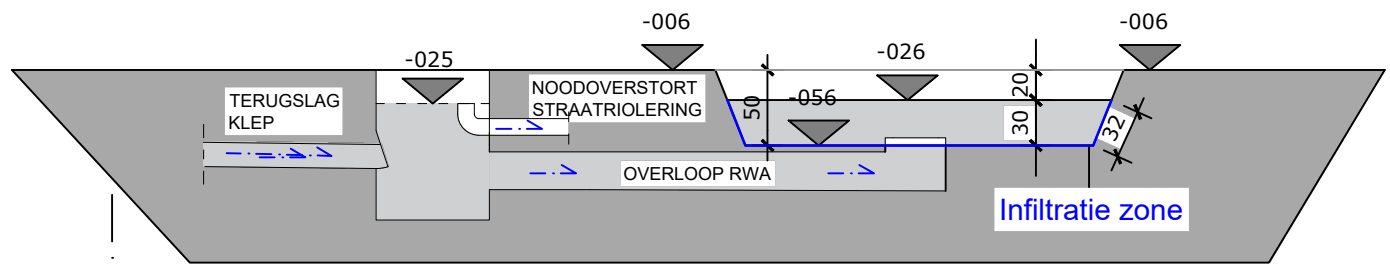
Principesnede Infiltratieput
