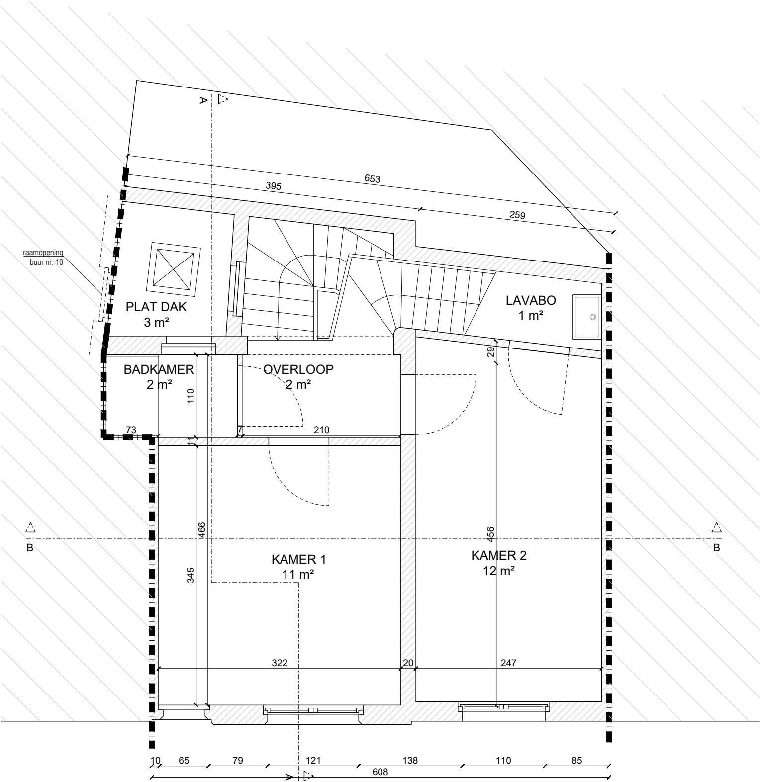
DUPLEXAPPARTEMENT NIVEAU 2 - BESTAAND
