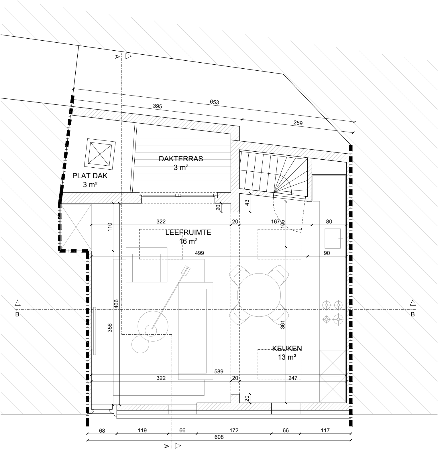
DUPLEXAPPARTEMENT NIVEAU 3
