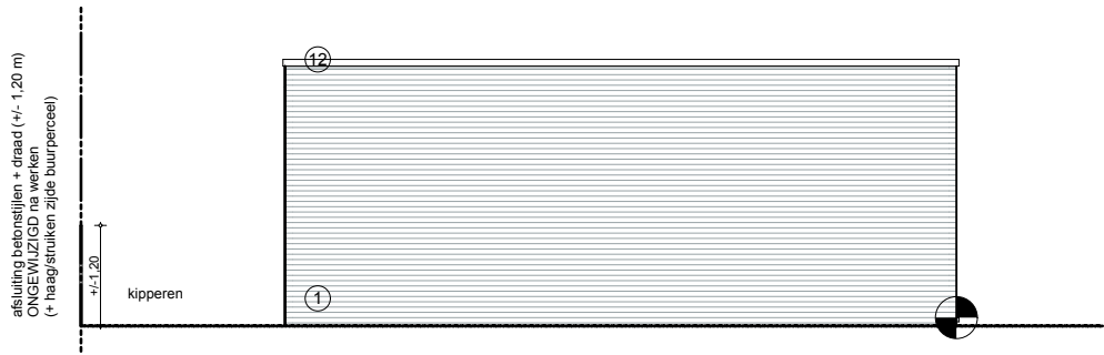
Zijgevel links bijgebouw Nieuwe toestand (ongewijzigd tov bestaand)
