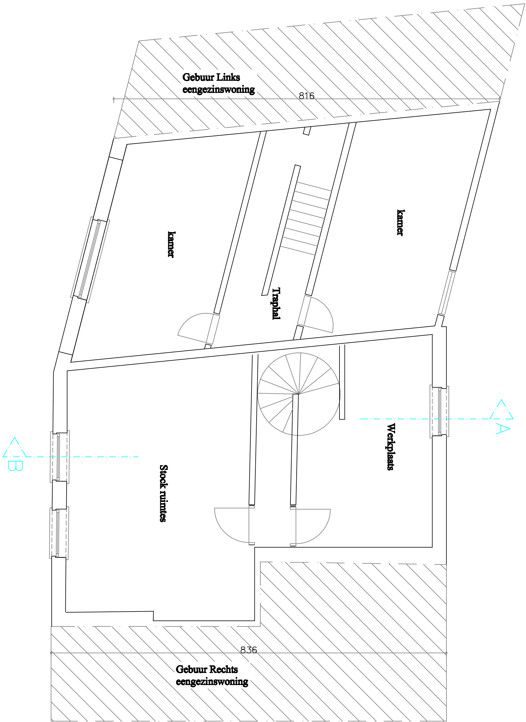
Eerste verdieping Bestaande toestand Schaal 1/50
