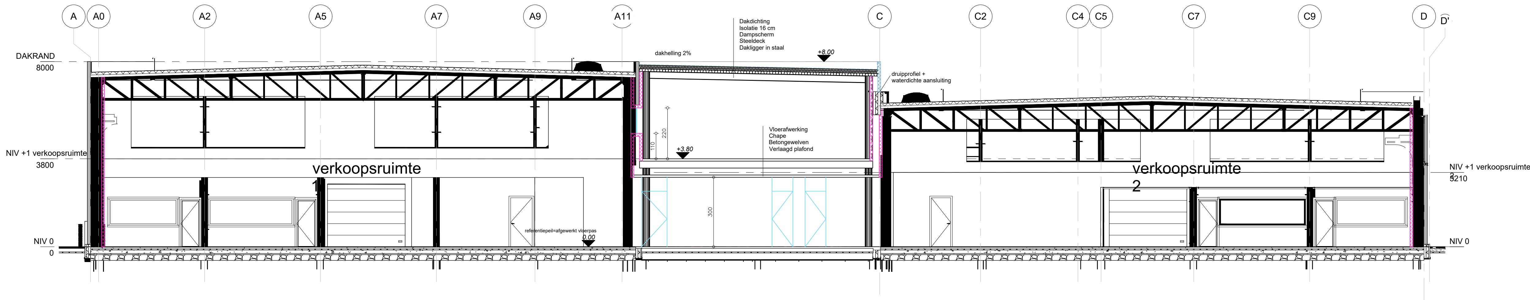
Doorsnede C-C'
