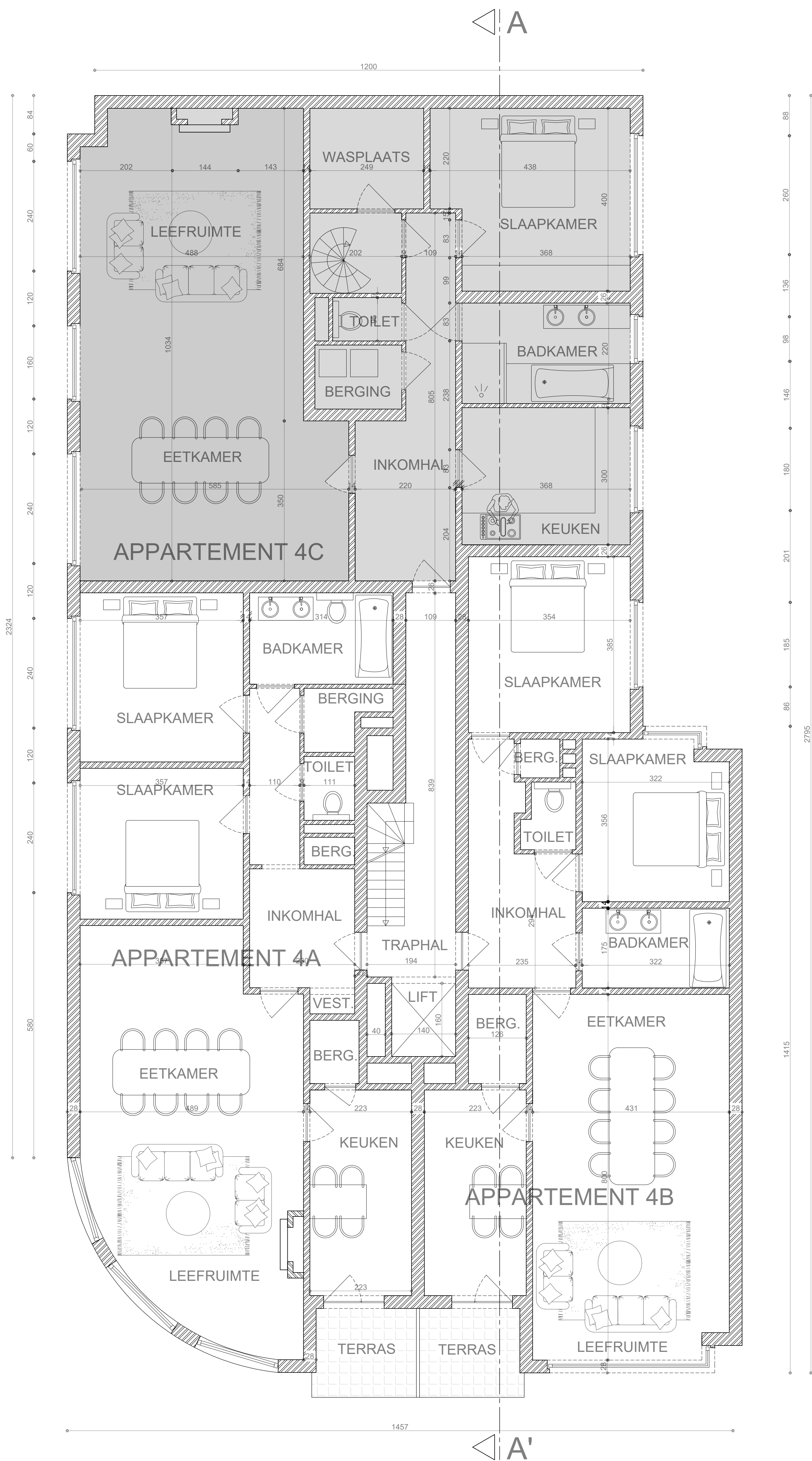
BESTAANDE TOESTAND app 4C GRONDPLAN 1/50 FLORALIENLAAN 48
