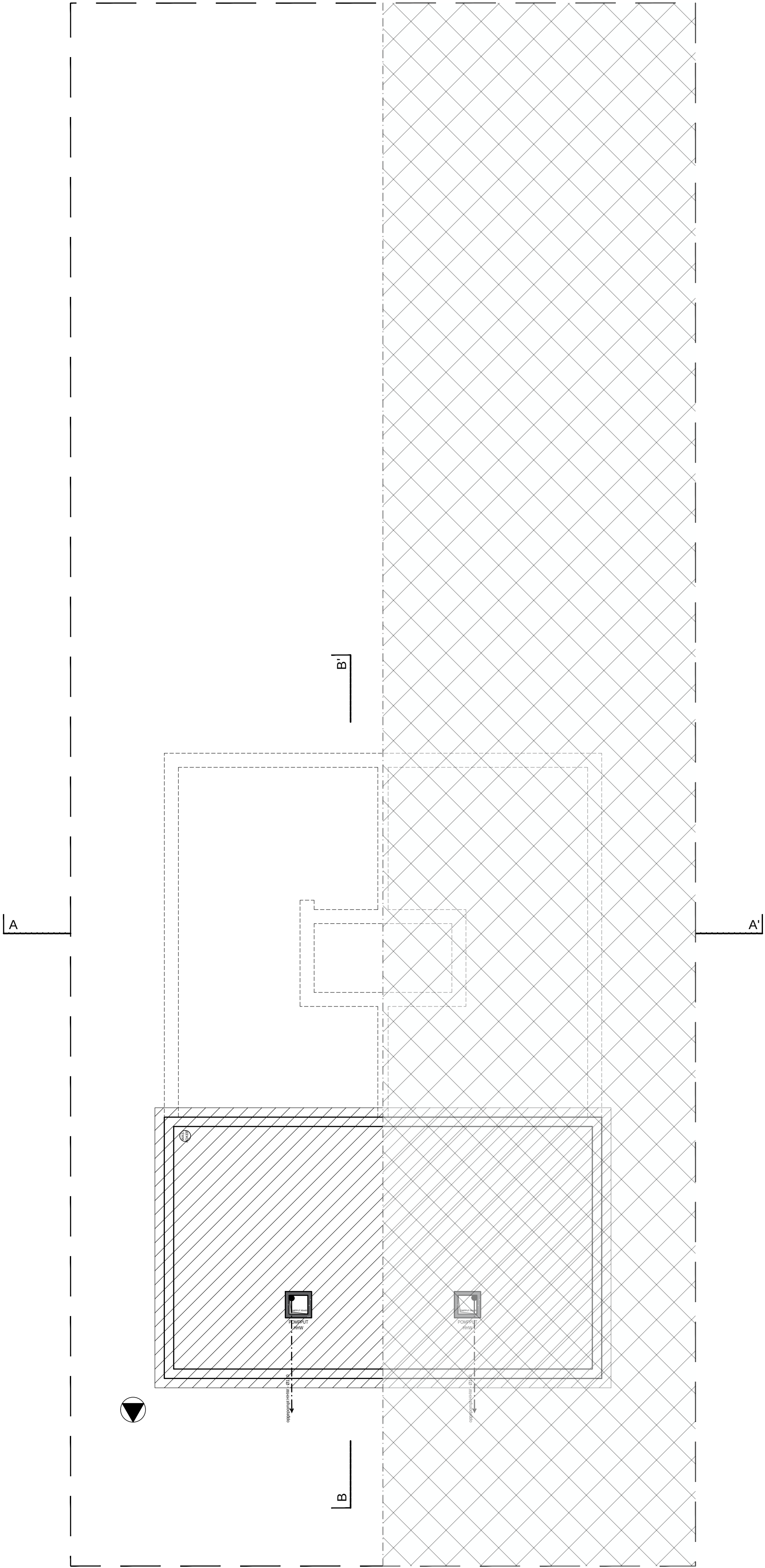
PLAN FUNDERINGS- EN RIOLERINGSSHEMA LOT 1
