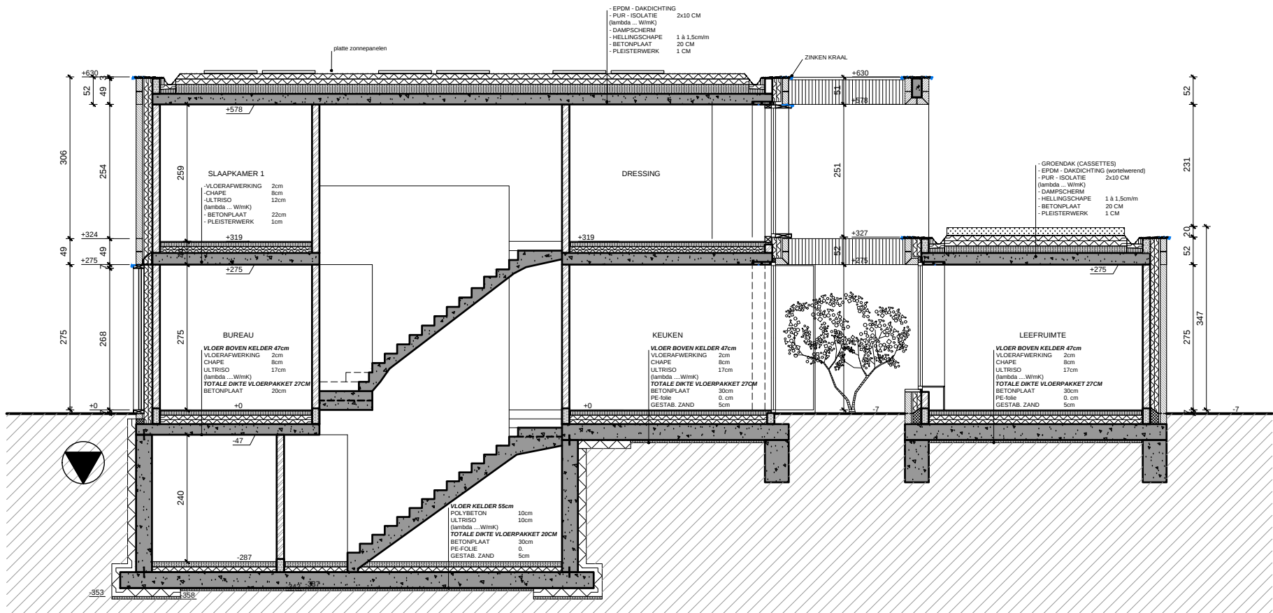
SNEDE BB'
