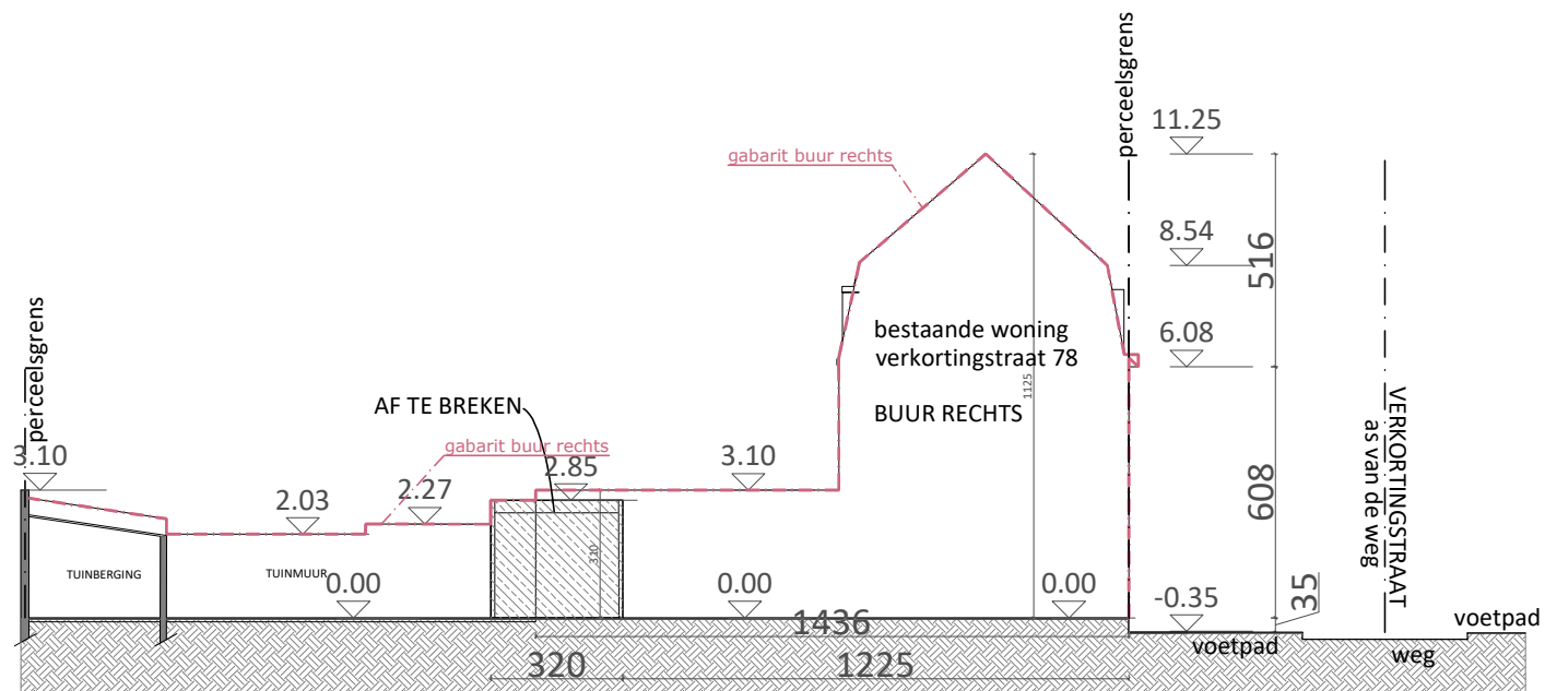
BESTAANDE TOESTAND BUUR RECHTS - TERREINPROFIEL B 1/200
