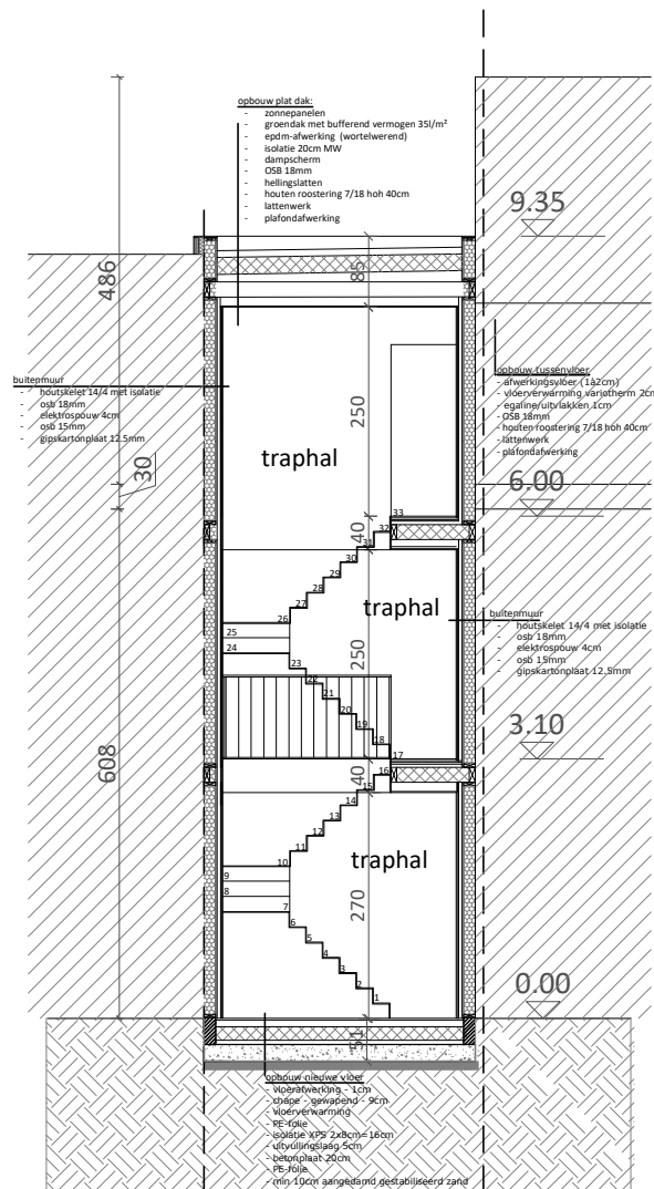
NIEUWE TOESTAND SNEDE D-D 1/100
