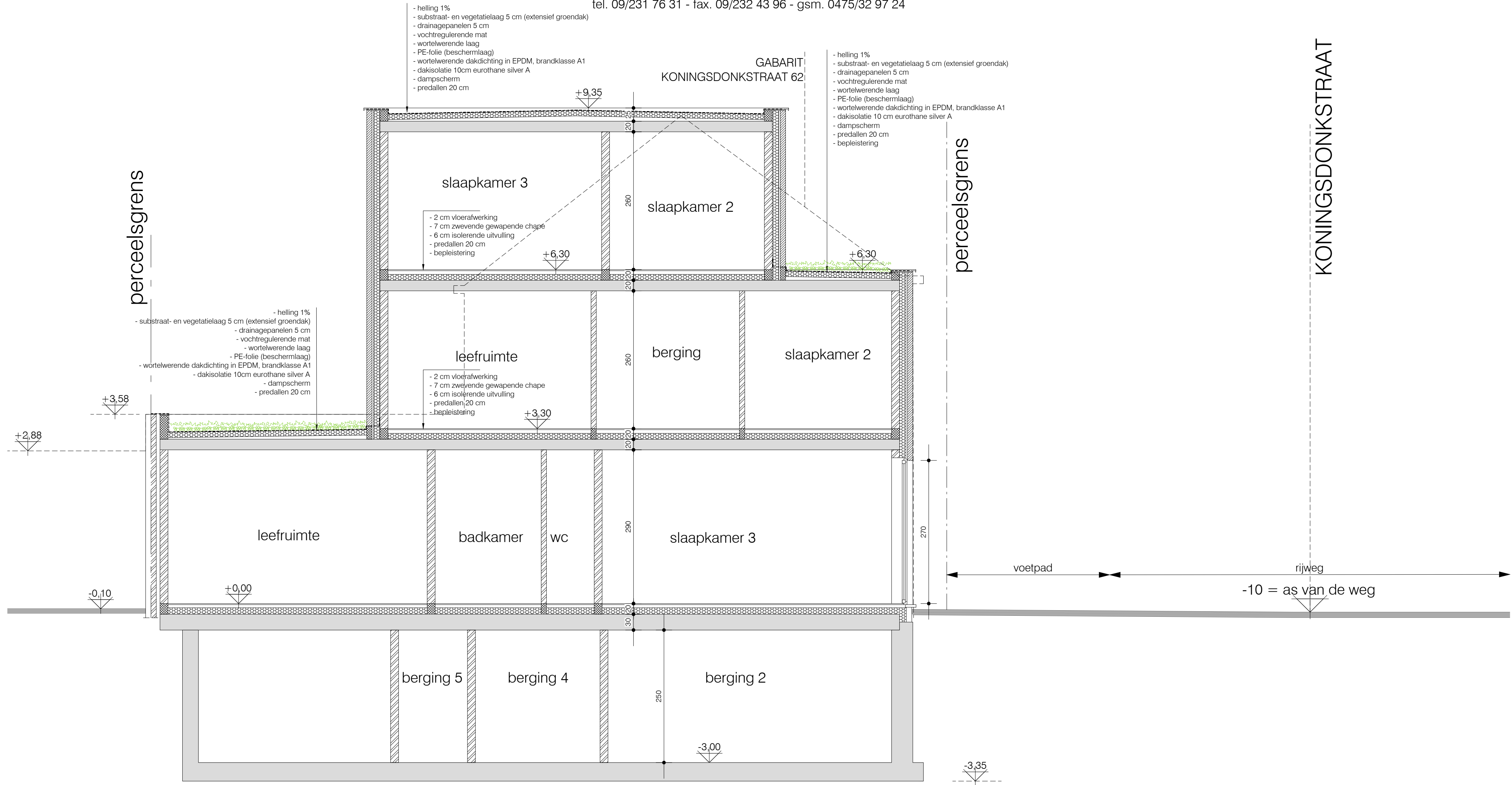
NIEUWE TOESTAND_SNEDE AA'
