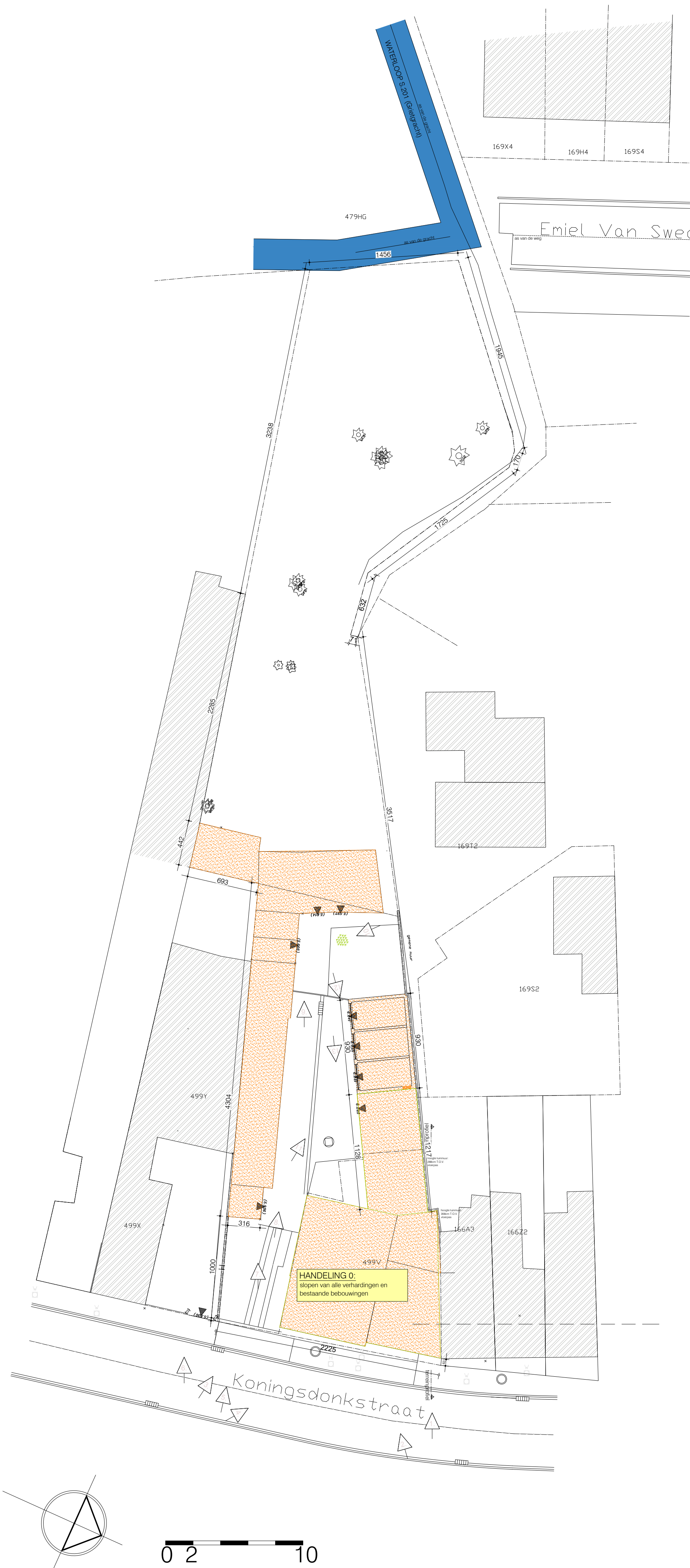
BESTAANDE TOESTAND_INPLANTINGSPLAN schaal: 1/200 - maatvoering in cm
