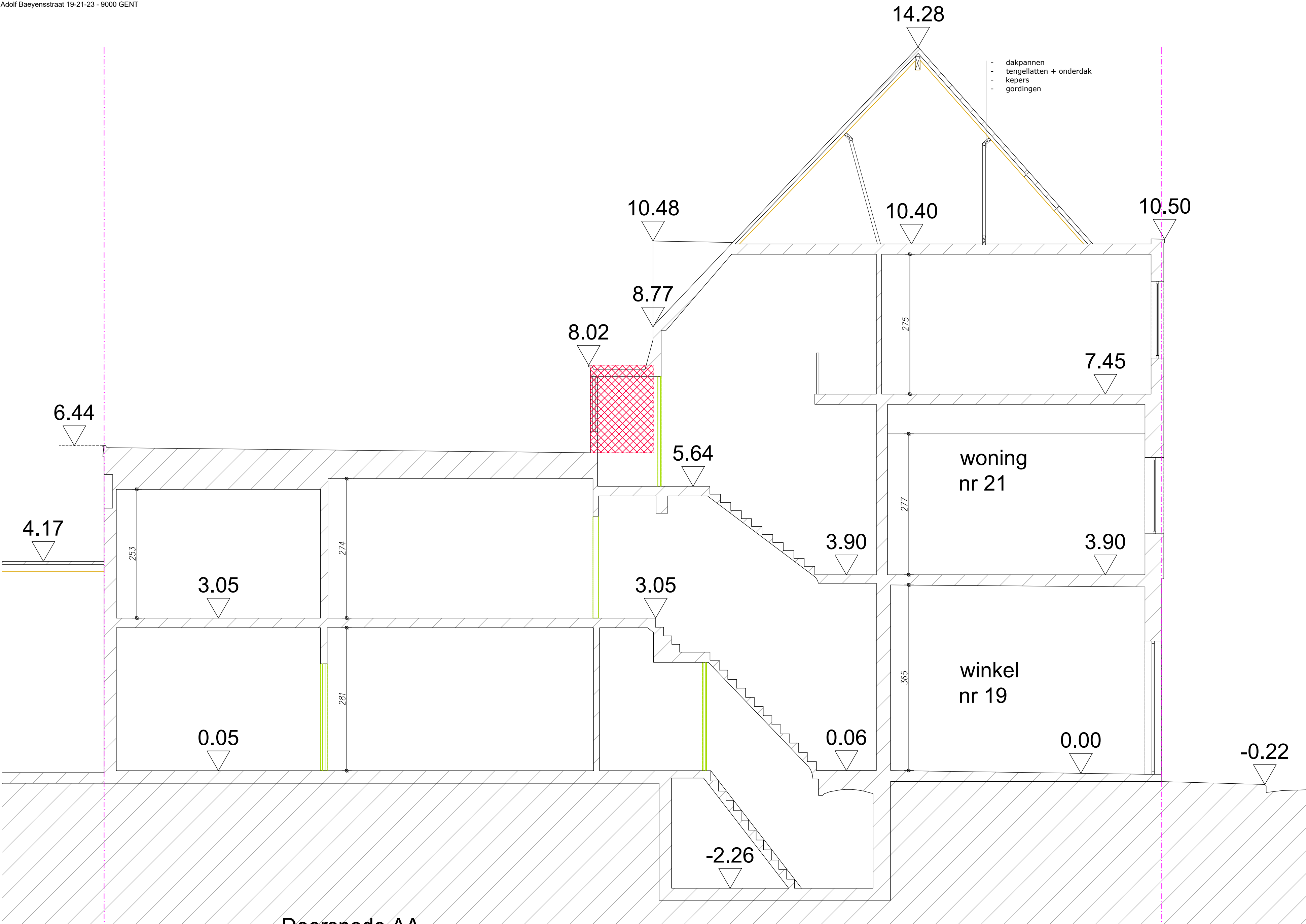
Doorsnede AA BESTAANDE TOESTAND
