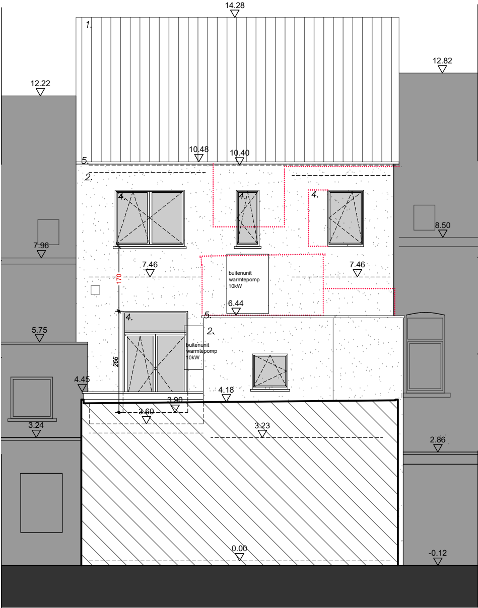
Gevel B (achtergevel woning)
