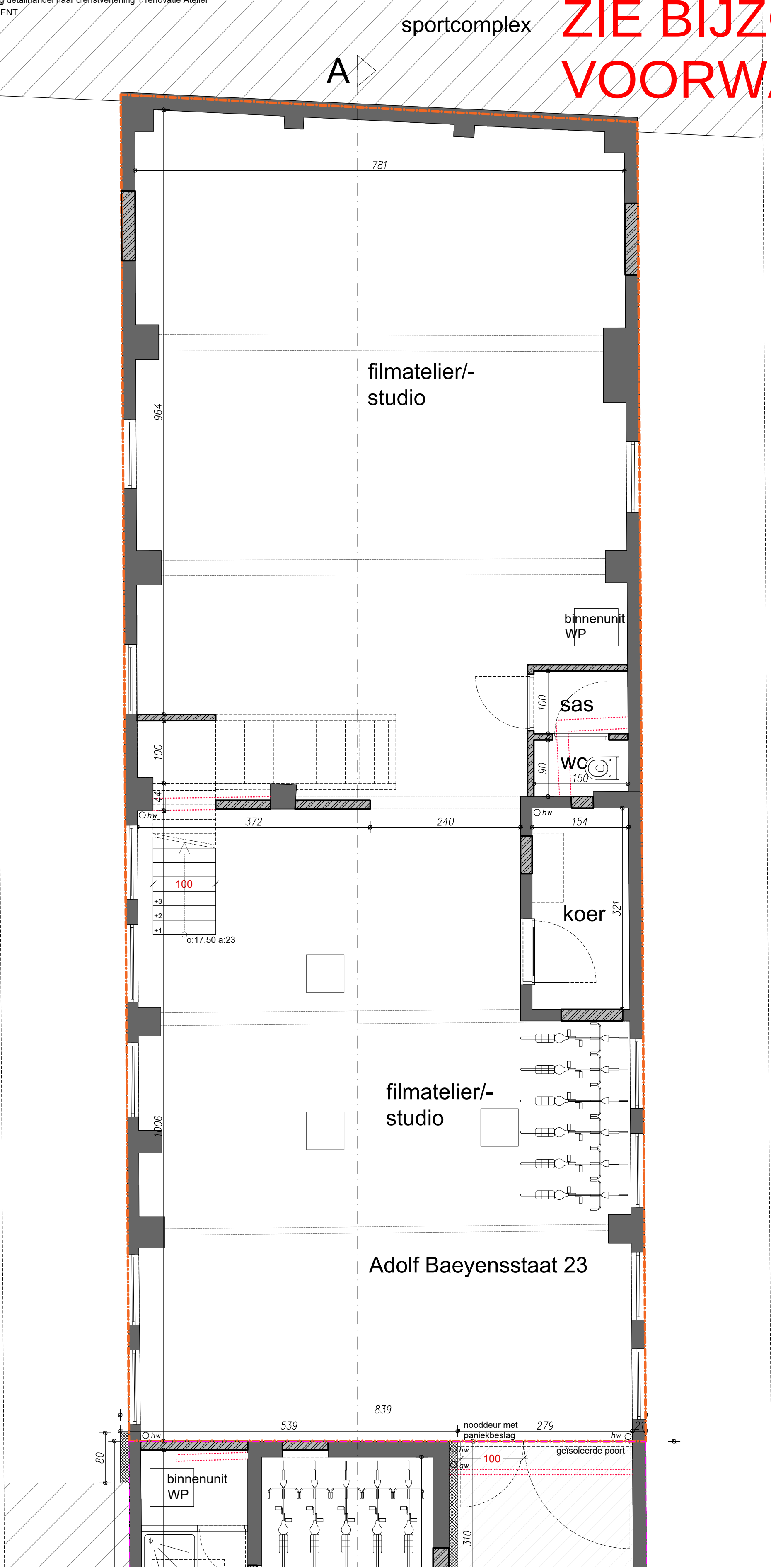
grondplan 0 NIEUWE TOESTAND
