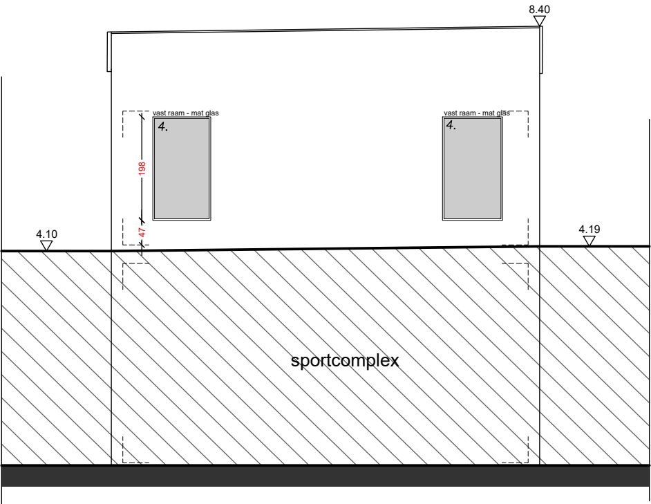
Gevel D (achtergevel atelier) NIEUWE TOESTAND
