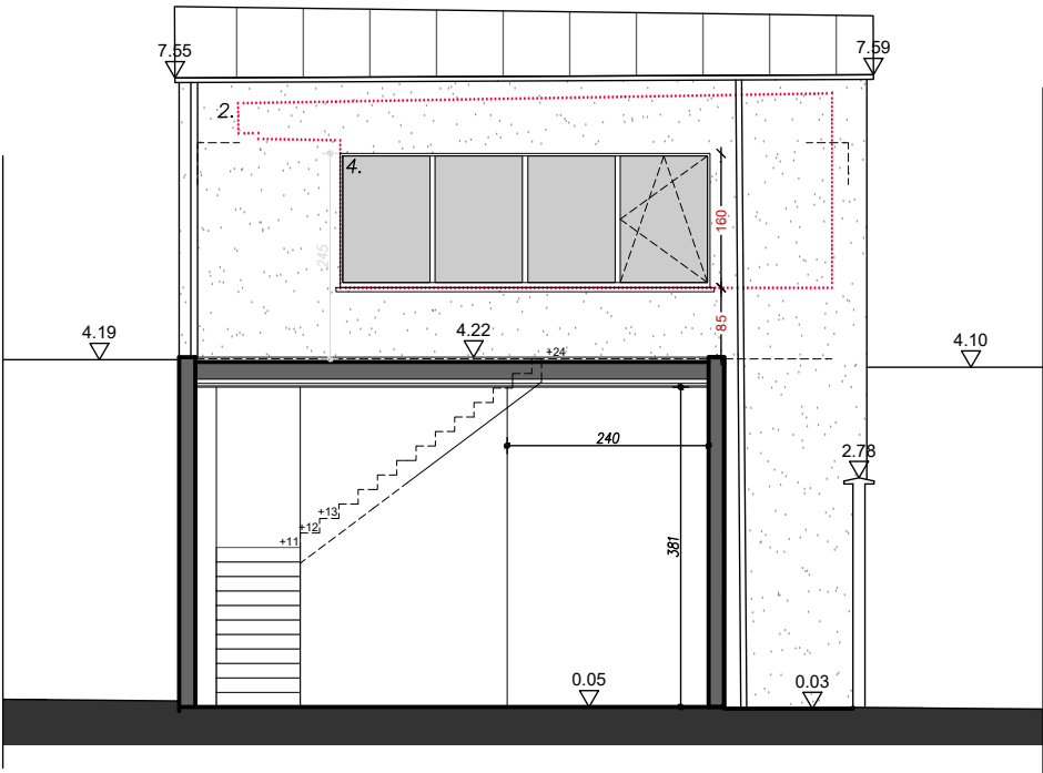
Gevel C (voorgevel atelier) NIEUWE TOESTAND
