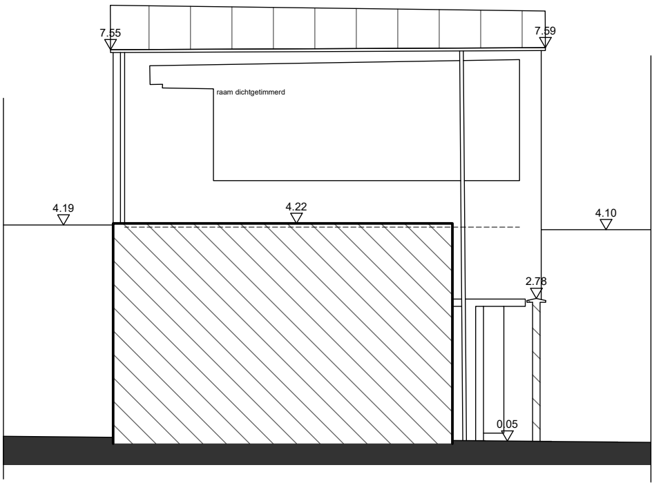
Gevel C (voorgevel atelier) BESTAANDE TOESTAND
