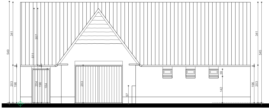
VOORGEVEL
