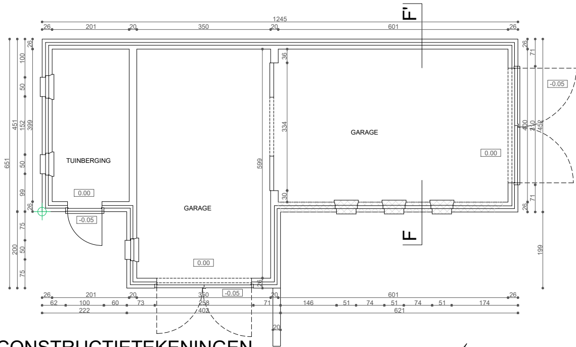
GRONDPLAN
