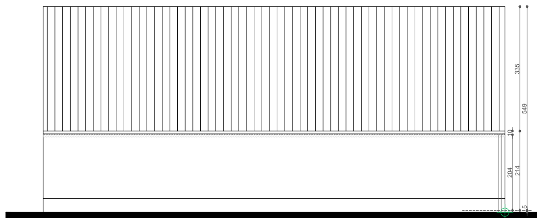
ACHTERGEVEL
