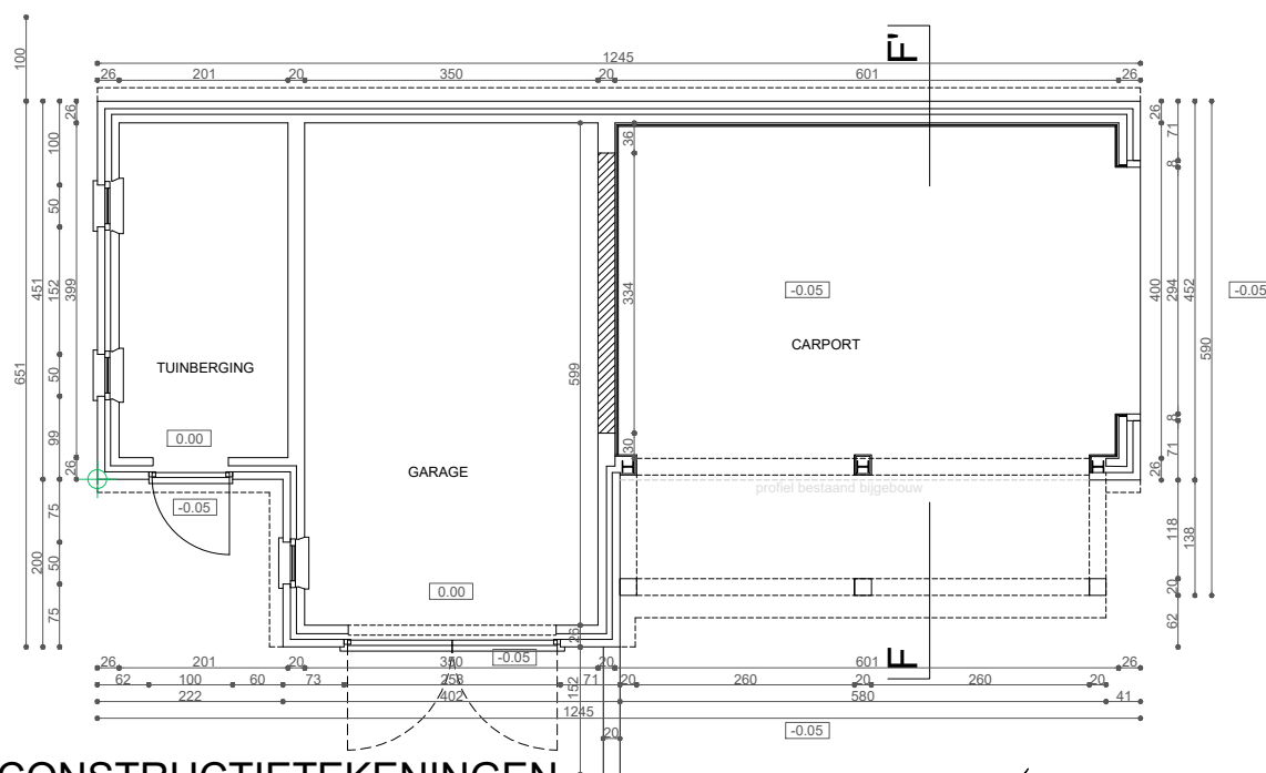
GRONDPLAN
