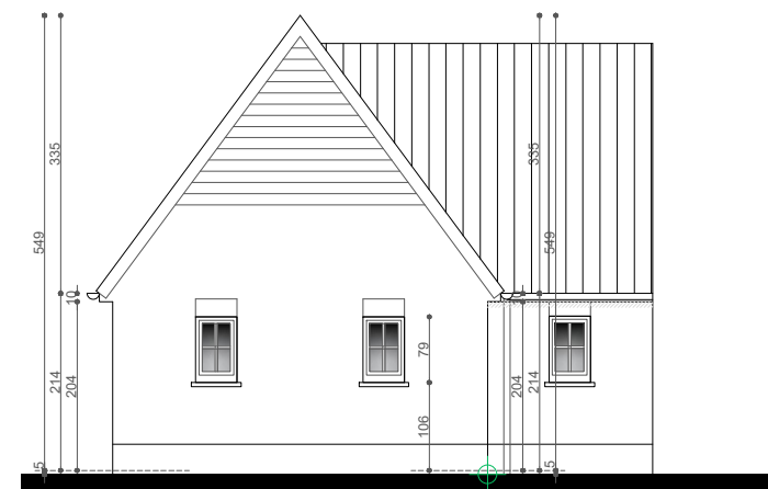
ZIJGEVEL LINKS
