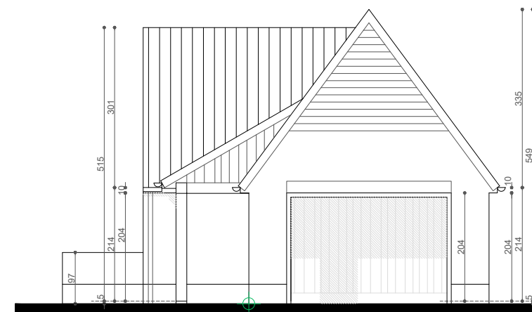
ZIJGEVEL RECHTS
