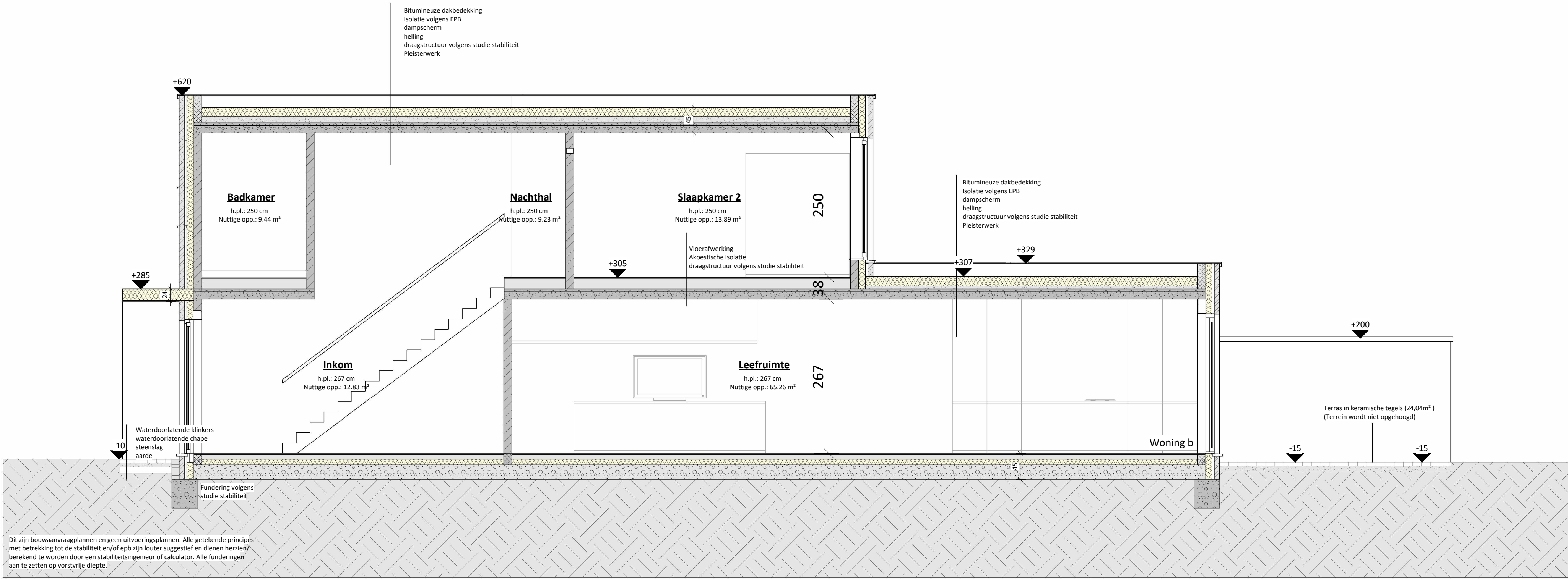
NT_Doorsnede CC | Nieuwe toestand | 1 : 50
