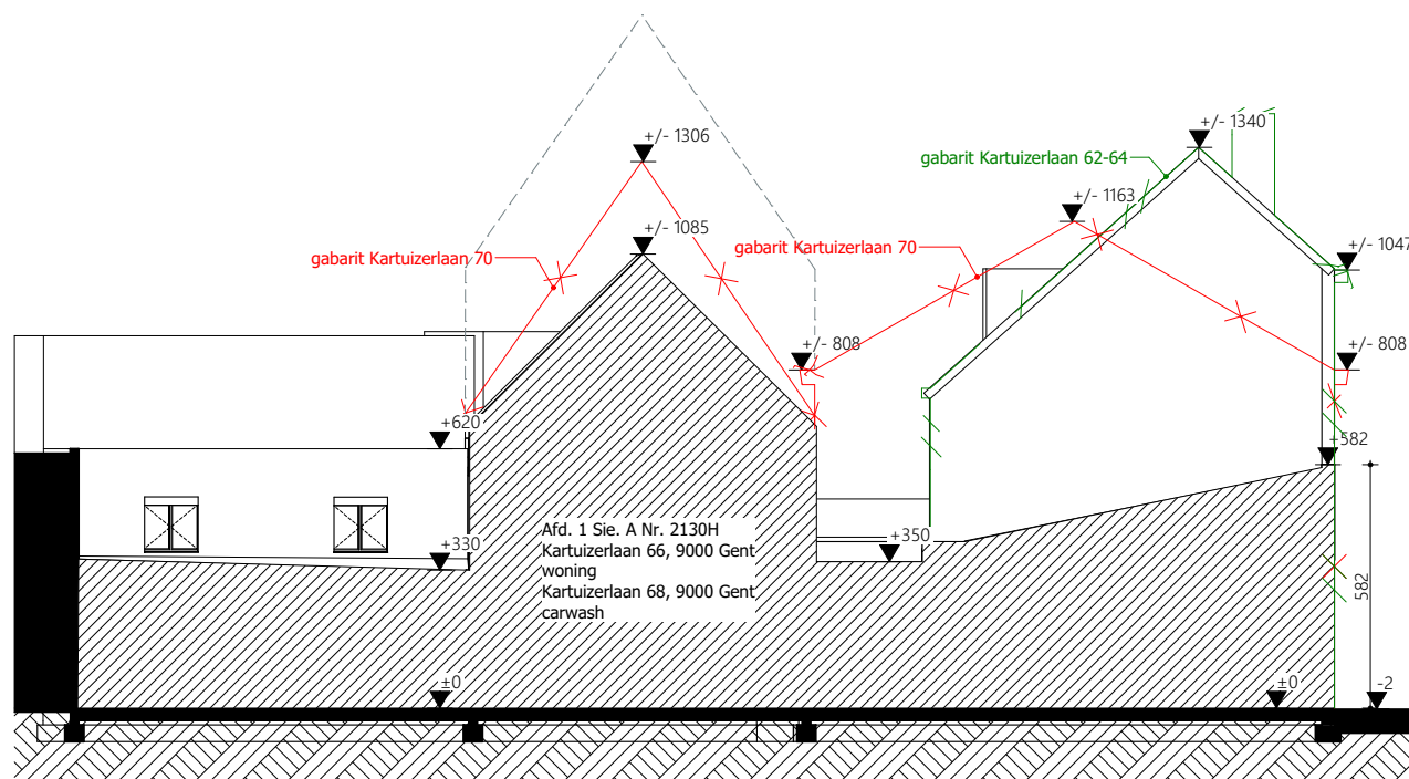
Terreinprofiel - nieuwe toestand
