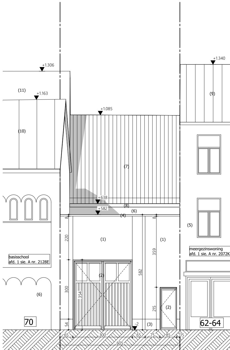
VG Voorgevel - nieuwe toestand 1:100
