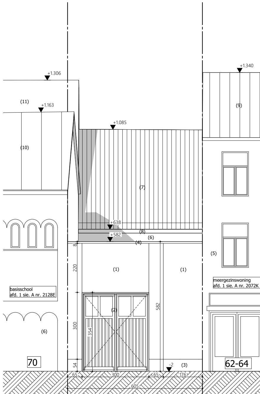
VG Voorgevel - bestaande toestand 1:100
