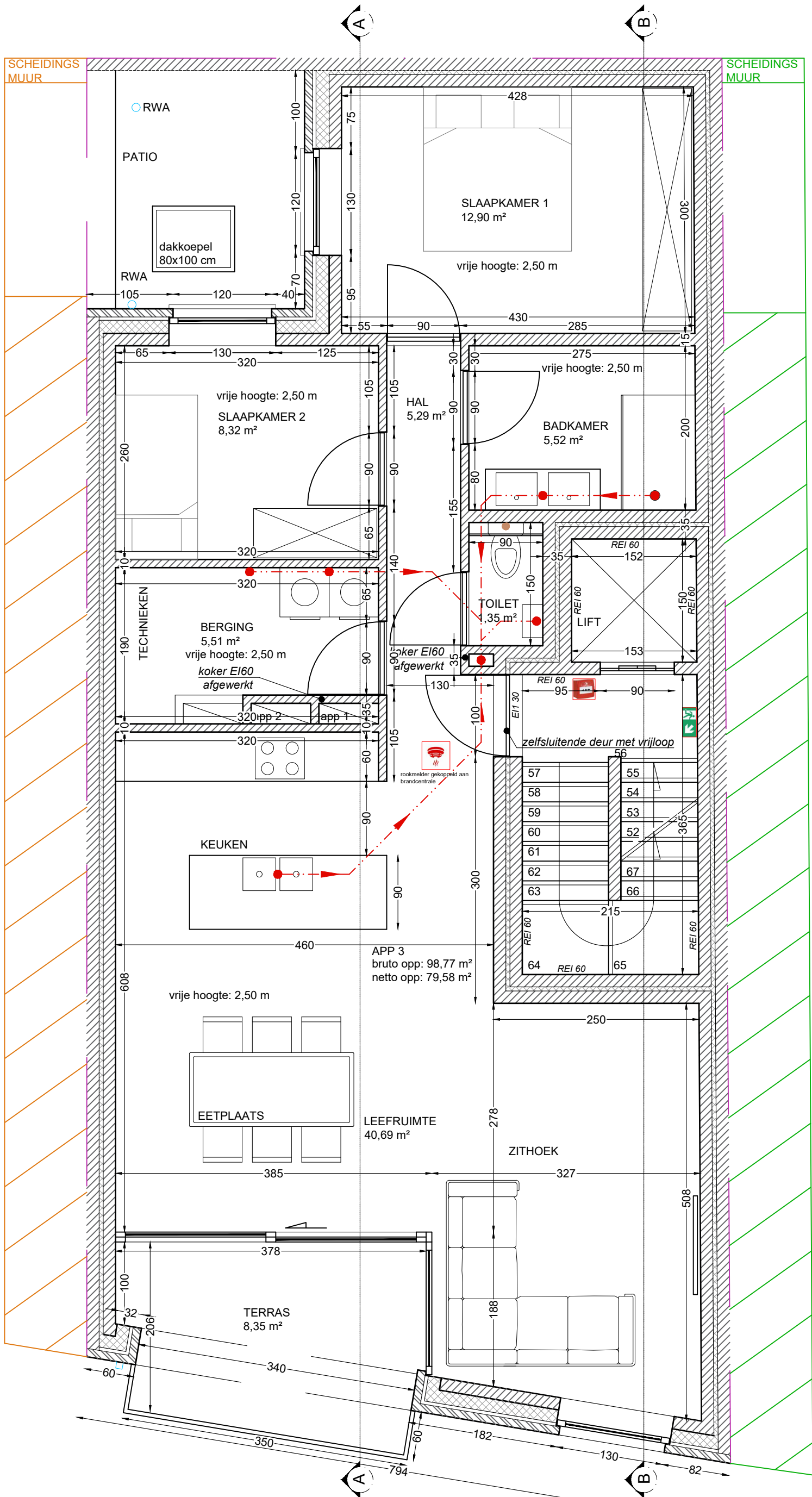
GRONDPLAN 3DE VERDIEP NIEUWE TOESTAND
