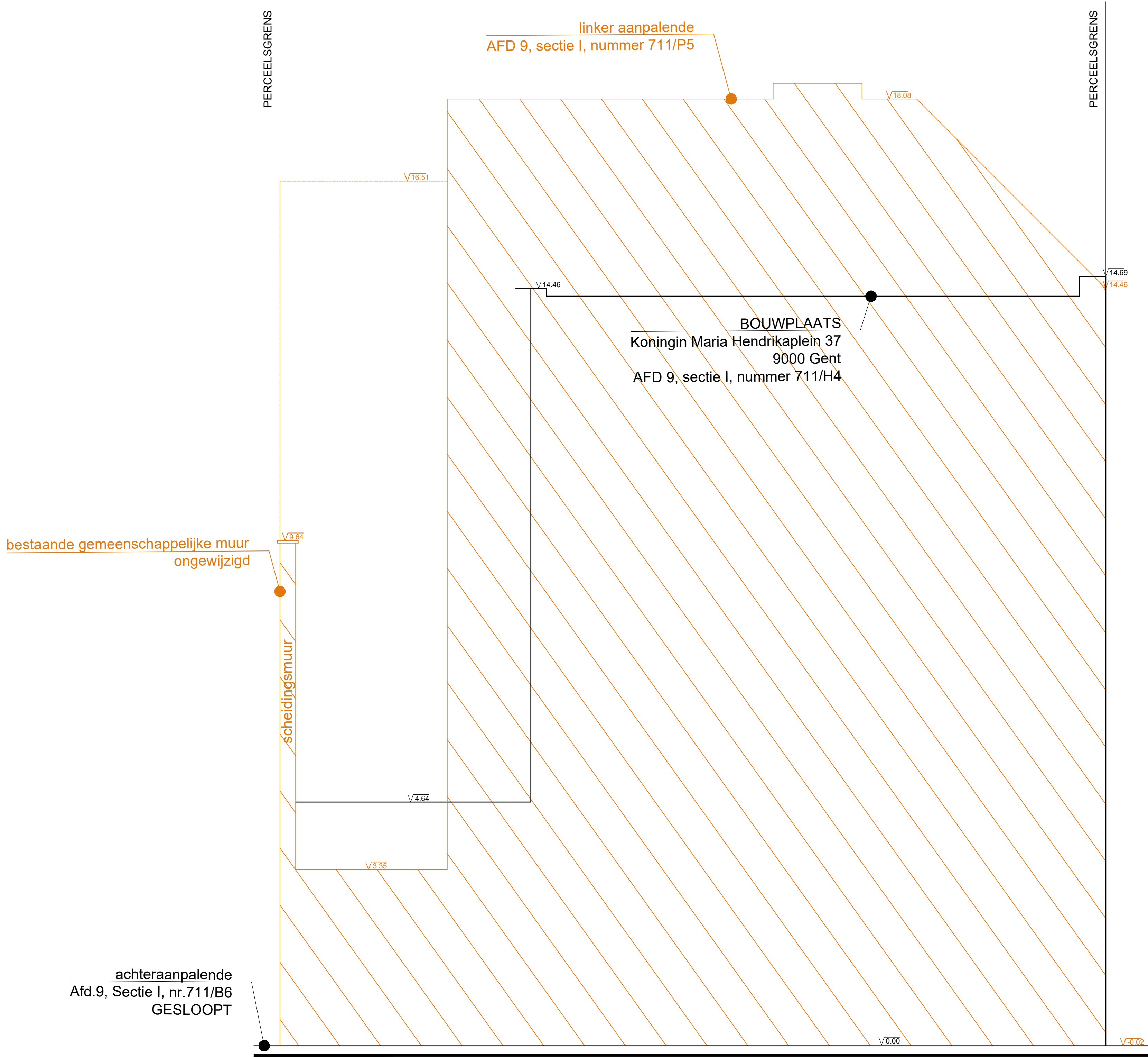
linkerzijgevel BESTAANDE TOESTAND
