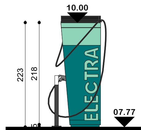
Zijaanzicht rechts: laadpaal HYC 400 kW Nieuwe toestand
