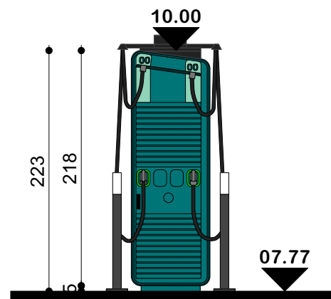
Vooraanzicht: laadpaal HYC 400 kW Nieuwe toestand
