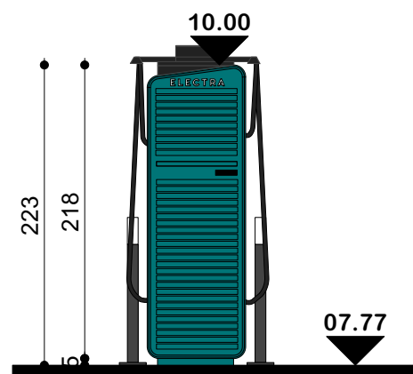
Achteraanzicht: laadpaal HYC 400 kW Nieuwe toestand
