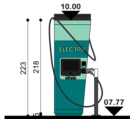
Zijaanzicht links: laadpaal HYC 400 kW Nieuwe toestand
