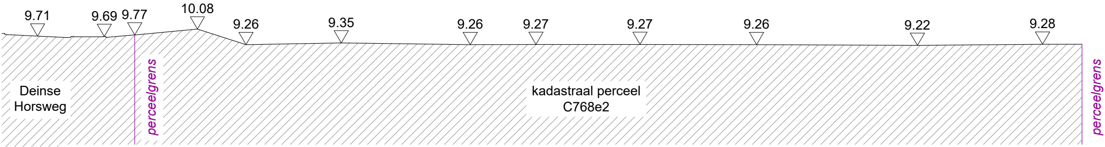
TERREINPROFIEL A
