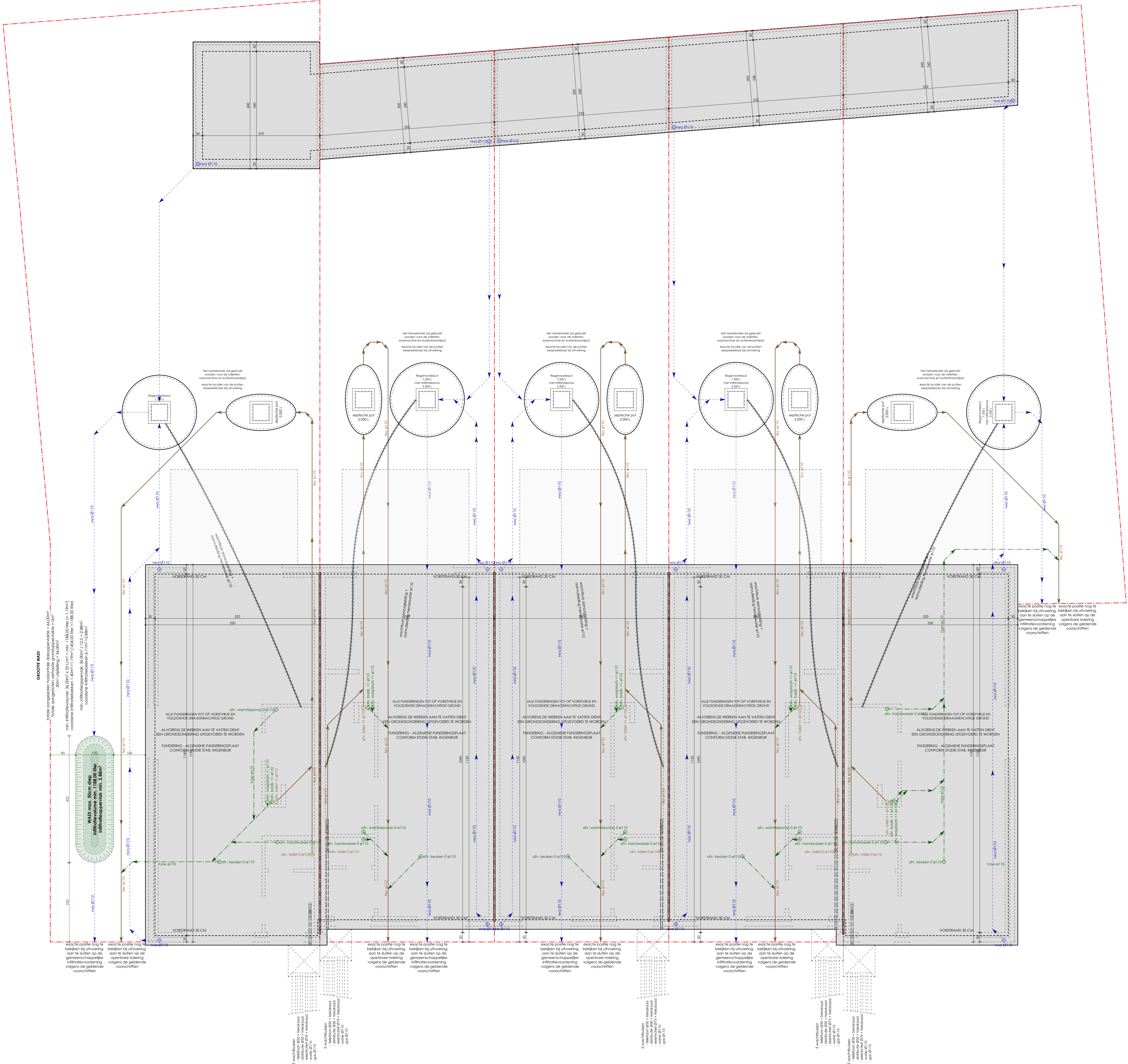
NT FUNDERINGS- EN RIOLERINGSPLAN schaal 1:50
