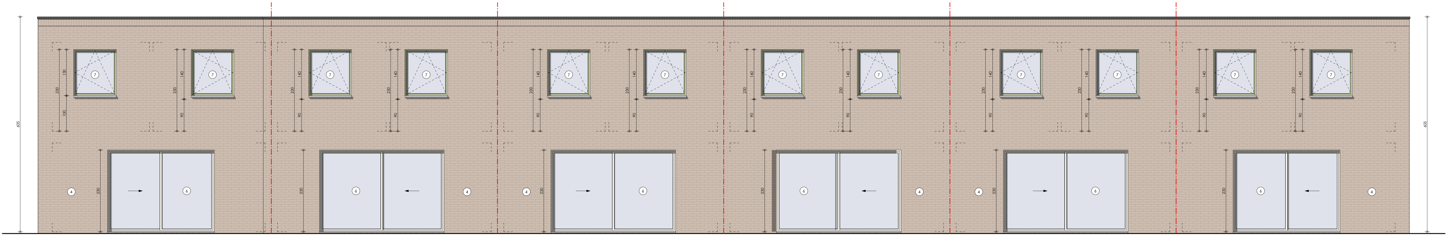
LOT 14 NT ACHTERGEVEL schaal 1:50 0 1 2m
