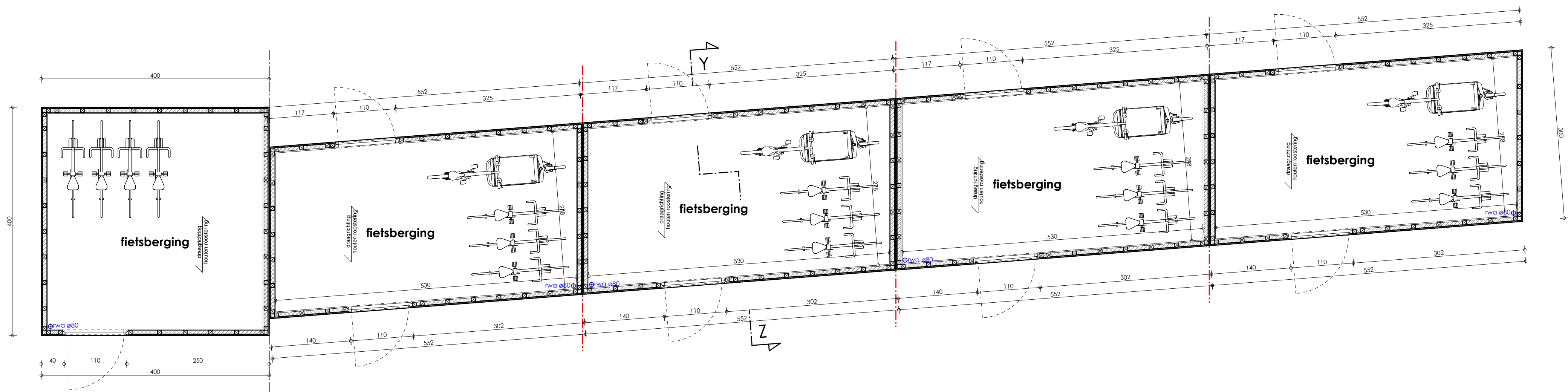
FIETSBERGING LOT 24 totale bruto opp: 13,21 m 2
