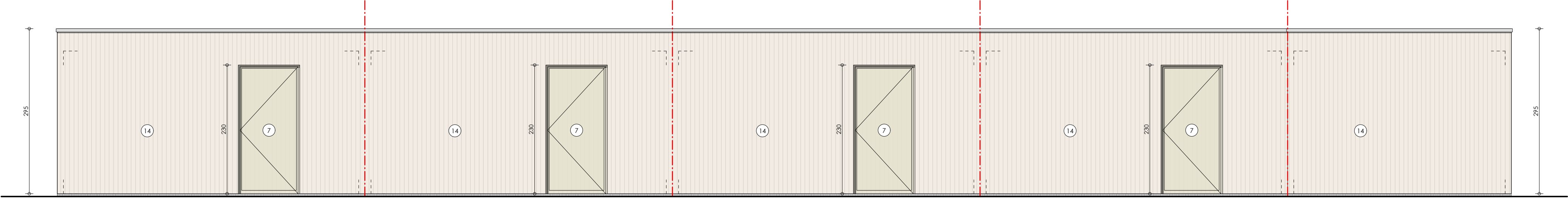
FIETSBERGING LOT 28 NT ACHTERGEVEL schaal 1:50 0 1 2m
