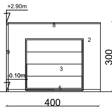
Voorgevel bijgebouw 1/100 NIEUWE TOESTAND
