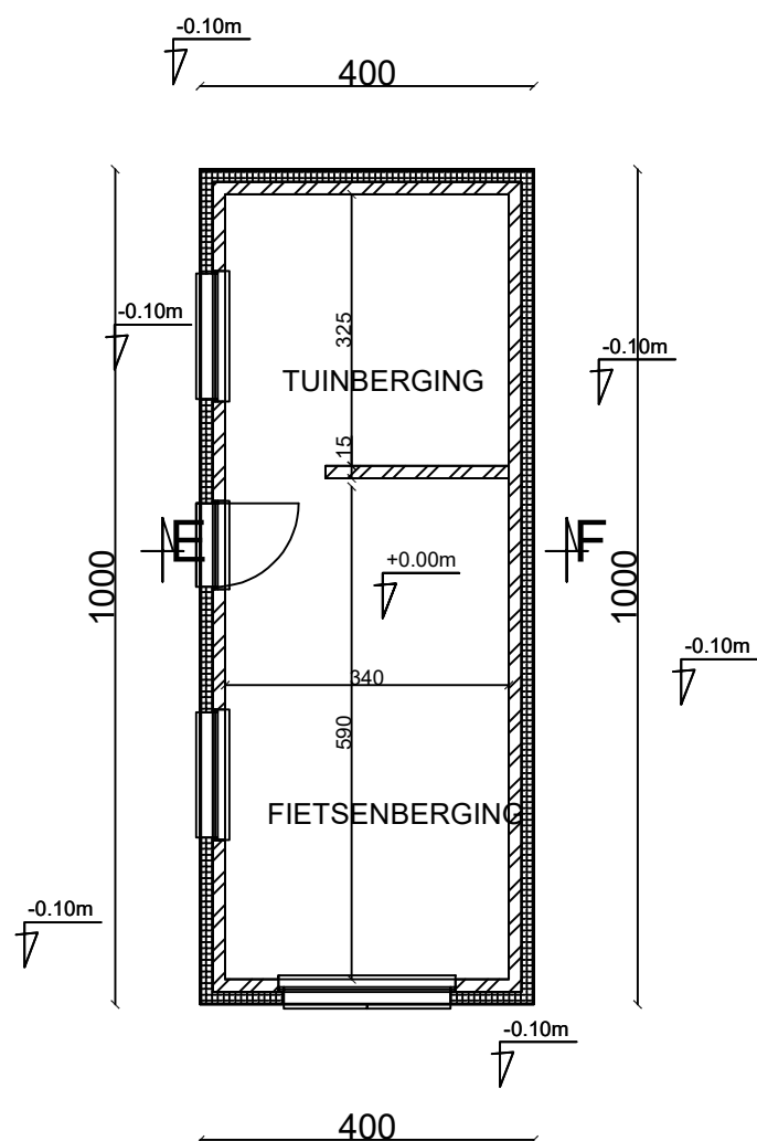
Grondplan bijgebouw 1/100 NIEUWE TOESTAND
